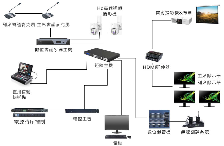
視聽環控系統架構圖
